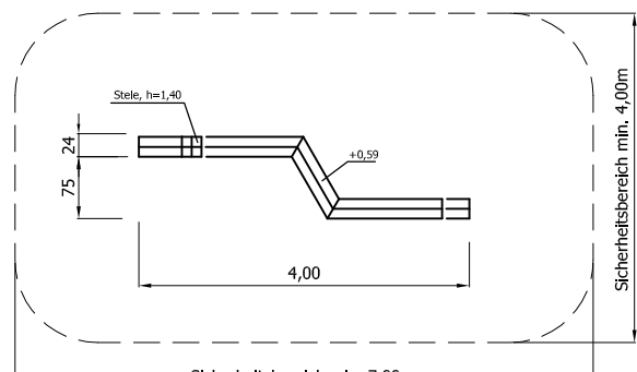
Draufsicht Typ 20 GAT 02 0420
