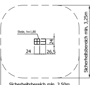
Draufsicht Typ 8 GAT 02 0408
