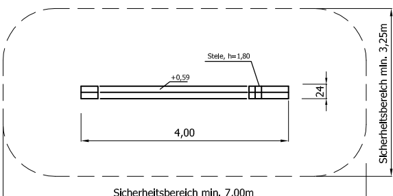
Draufsicht Typ 10 GAT 02 0410
