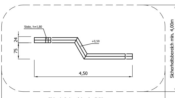
Draufsicht Typ 21 GAT 02 0421
