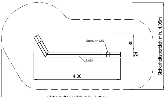
Draufsicht Typ 17 GAT 02 0417
