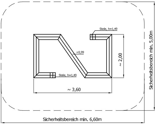
Draufsicht Typ 3 GAT 02 0403
