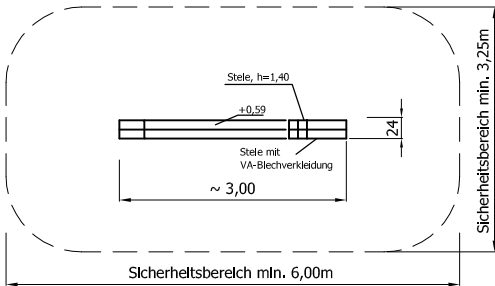
Draufsicht Typ 7 GAT 02 0407
