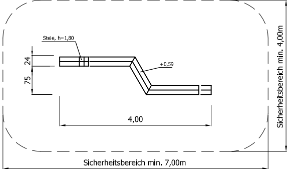
Draufsicht Typ 13 GAT 02 0413
