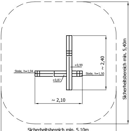
Draufsicht Typ 2 GAT 02 0402
