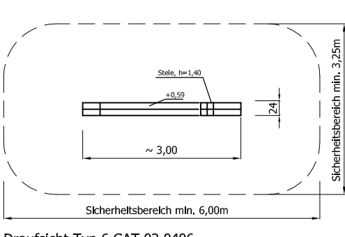
Draufsicht Typ 6 GAT 02 0406
