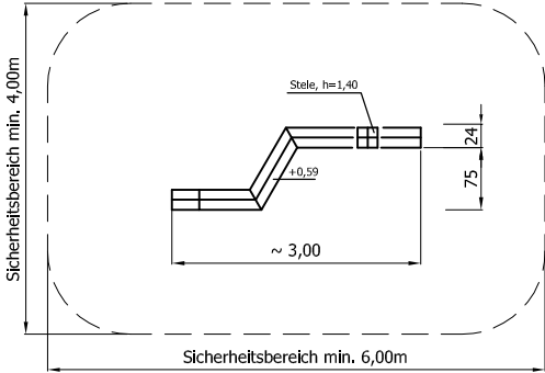
Draufsicht Typ 5 GAT 02 0405
