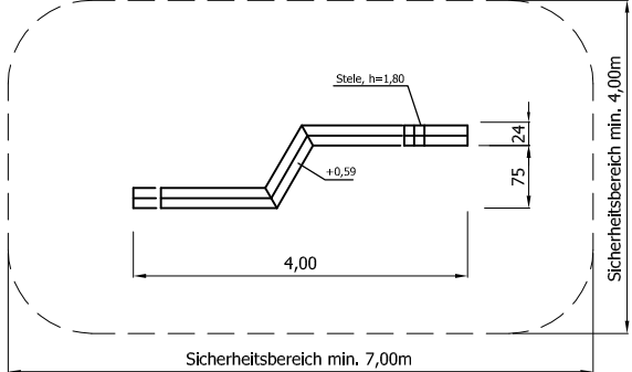
Draufsicht Typ 12 GAT 02 0412
