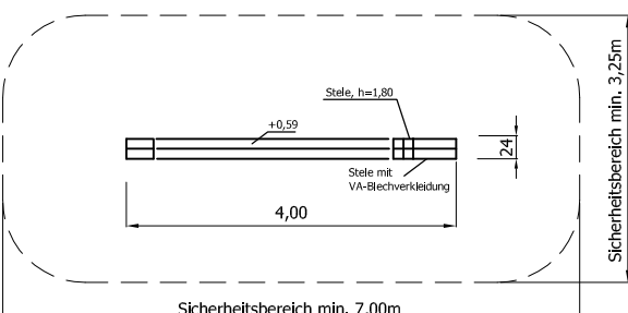
Draufsicht Typ 11 GAT 02 0411
