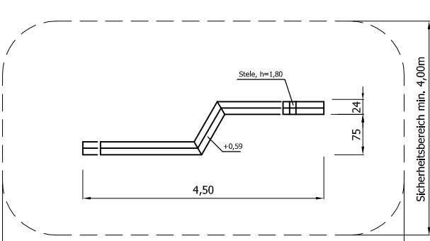
Draufsicht Typ 19 GAT 02 0419
