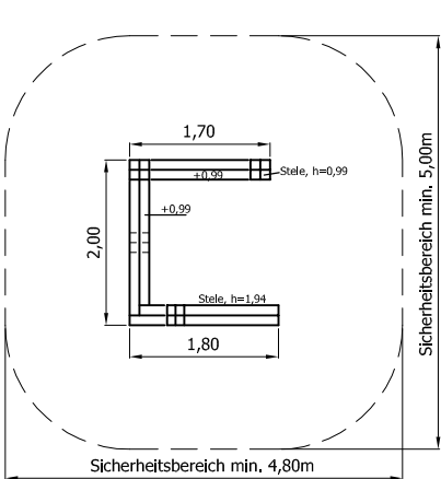
Draufsicht Typ1 GAT 02 0401
