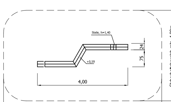
Draufsicht Typ 18 GAT 02 0418
