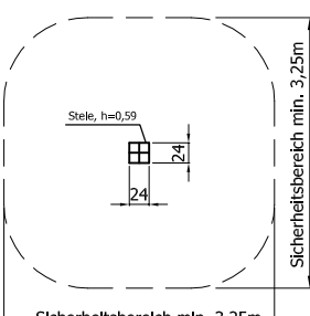
Draufsicht Typ 9 GAT 02 0409
