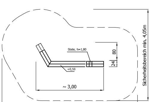
Draufsicht Typ 16 GAT 02 0416
