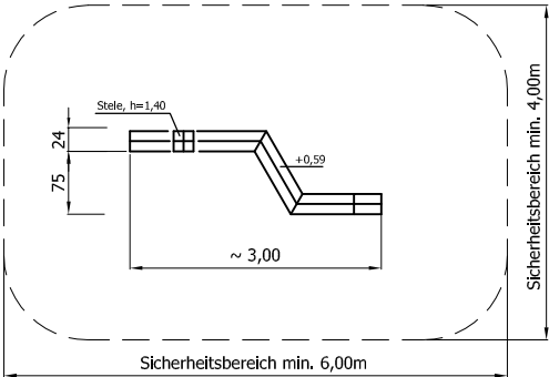
Draufsicht Typ 4 GAT 02 0404
