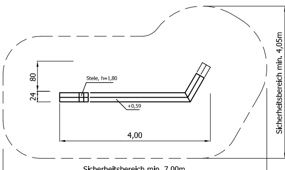
Draufsicht Typ 15 GAT 02 0415
