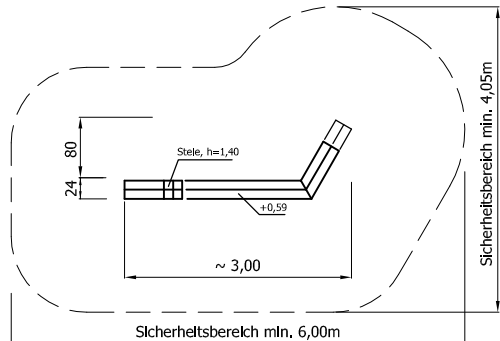
Draufsicht Typ 14 GAT 02 0414
